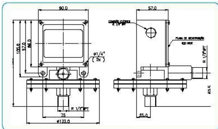
DESENHO DIMENSIONAL
